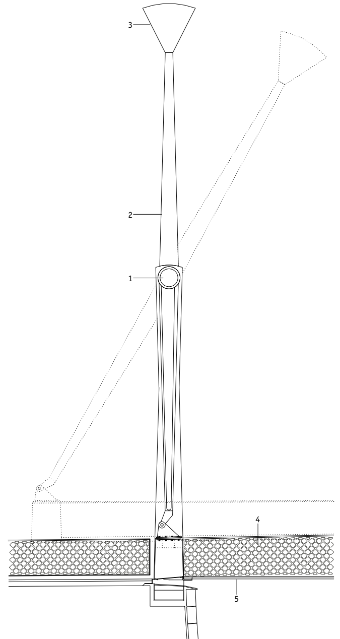
Longitudinal section, 1:100
